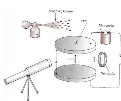
Πείραμα Millikan
